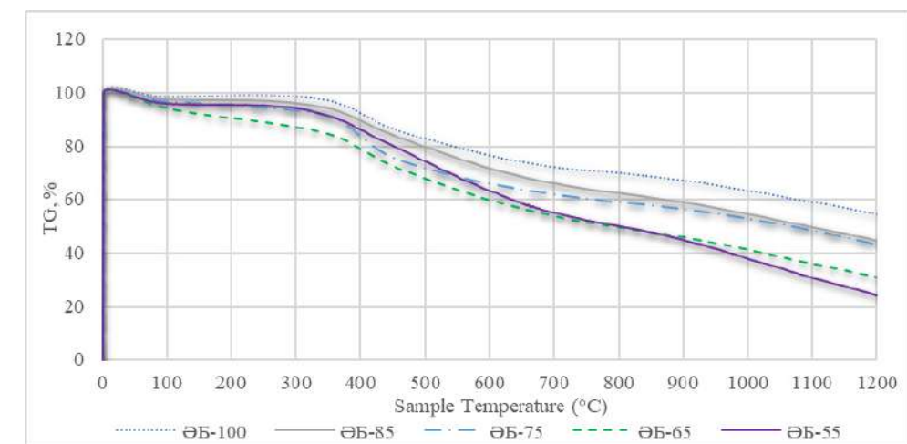
1-сурет – Зерттелетін үлгілердің массасының жоғалуы
