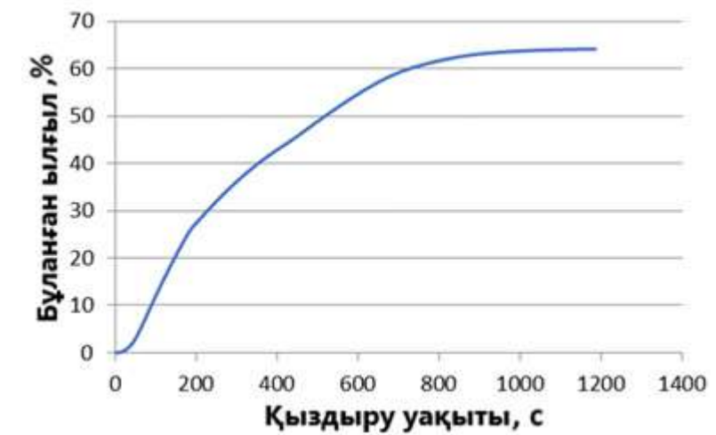
7-сурет – Экспресс-қыздыру арқылы майлылығы 2 % сүзбеден ылғалдың булануы
