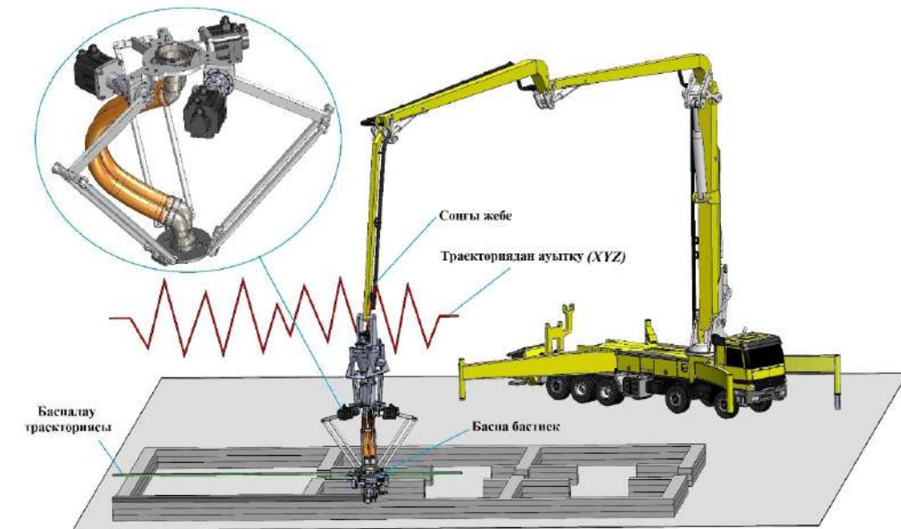
1-сурет – Басып шығару процесінде дәл позициялау үшін қажетті қозғалыстарды анықтау
