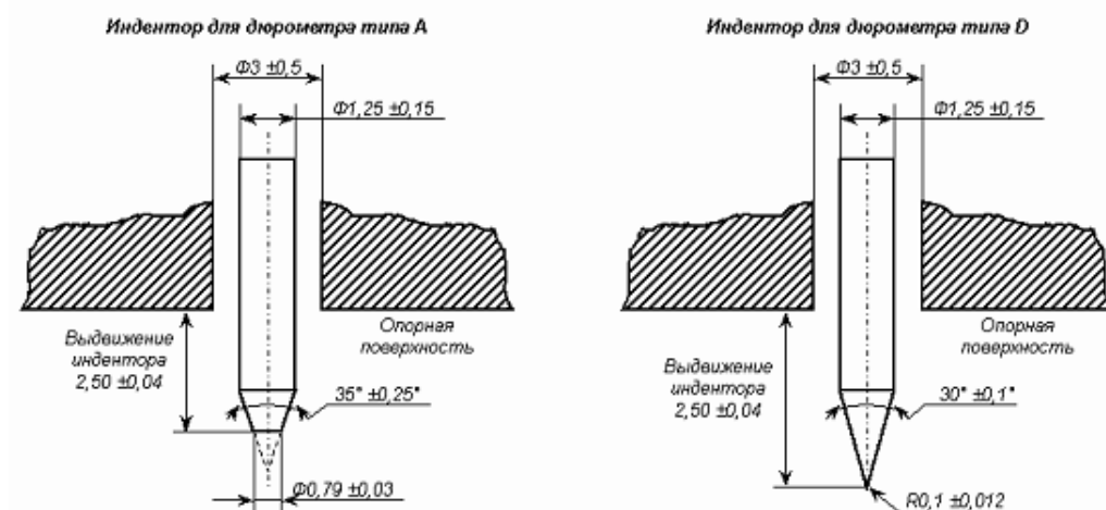
2-сурет – А және D типті дюрометрлерге арналған индендорлардың сызбалары
