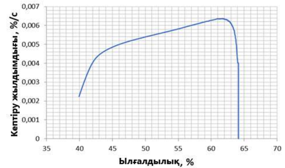
6-сурет – Майлылығы 2% сүзбені кептіру жылдамдығының қисығы
