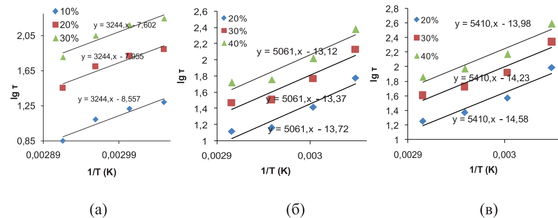
Рисунок 6 – Кинетика выщелачивания Pb (а), Cu (б) и Zn (в) в водном растворе HCl
