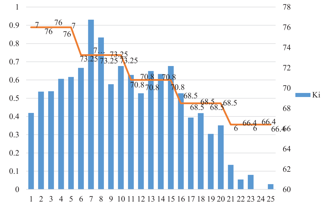
8 – сурет – Қож ваннасындағы кернеудің балқытылған тістер сапасының кешенді көрсеткішіне әсері
