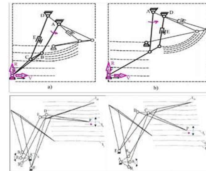
Рисунок 1 – Схемы реконфигурируемых четырехзвенных механизмов: ABCDE – шарниры; R – реакция ноги; P – точка шатуна; t_1, t_2, t_4, t_5, t_{10} – линии траектории (позиционное движение); V – скорость ноги
