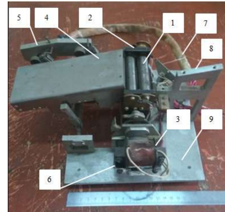
Рисунок 3 – Прибор для контроля некруглости и РСЦМ
