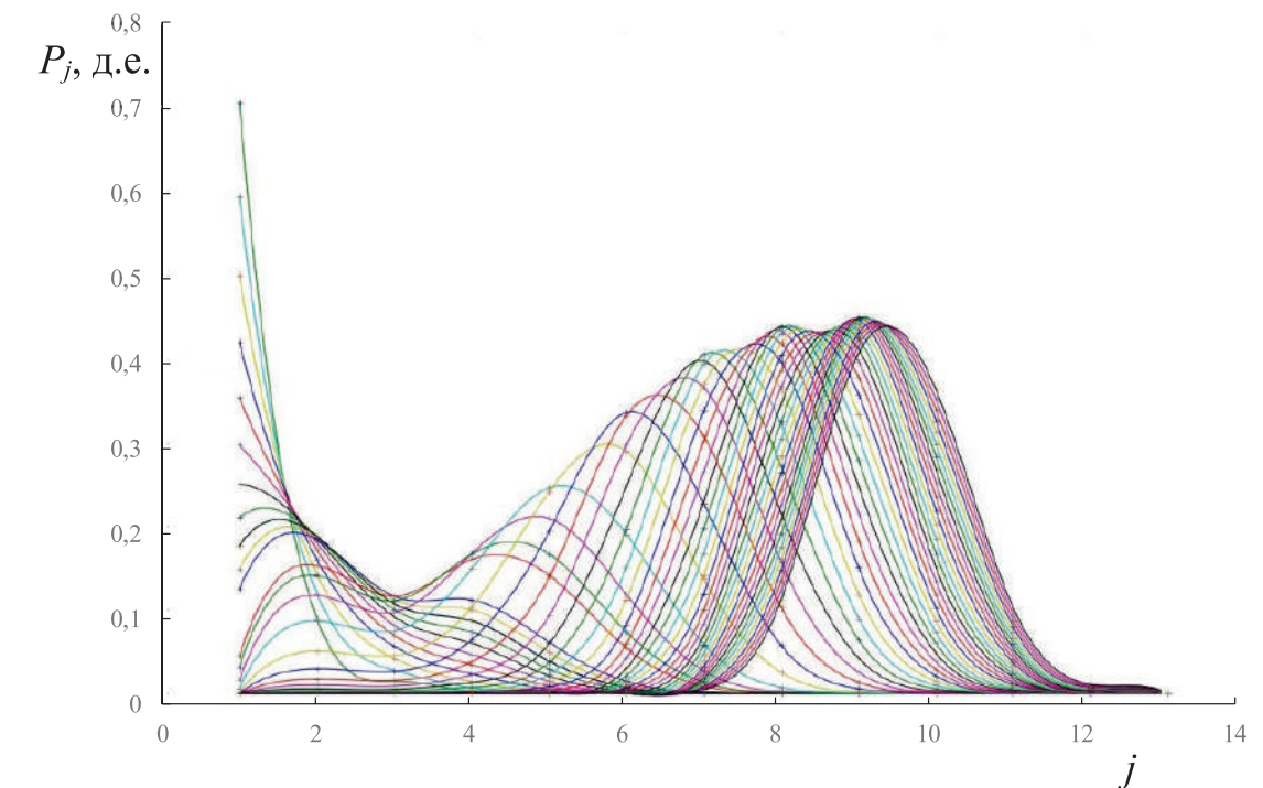
Рисунок 2 – Зависимость фракционного состава от кратности и продолжительности измельчения по интегральной модели (3).
