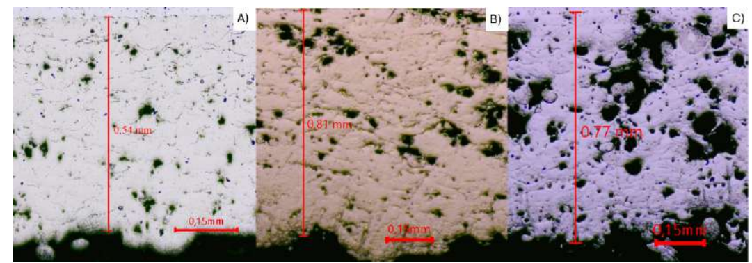
Рисунок 3 – Значения измерения толщины покрытий а) нагрев в печи б) нагрев пистолетом с) исходное покрытие
