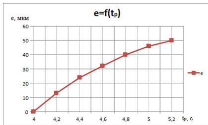
Рисунок 2 – Зависимость РСЦМ от времени разгона
