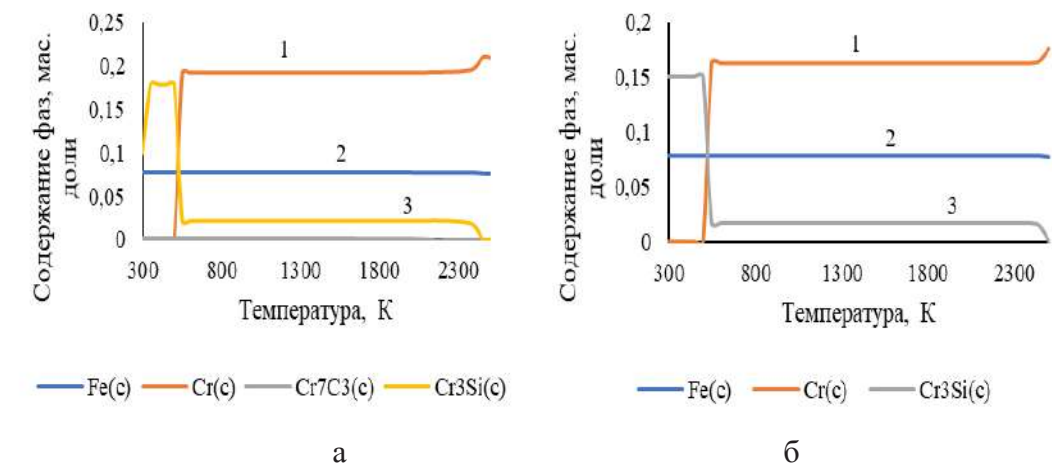
Рисунок 5 – Динамика изменения фазового состава основного металла с температурой по заводской технологии (а) и с применением комплексного ферросплава ФАСК (б).
