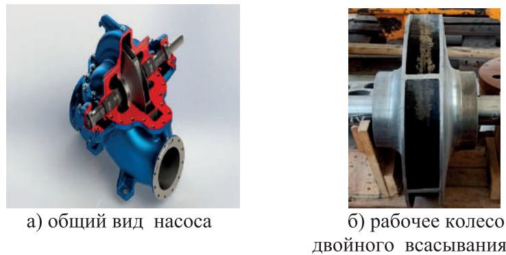
Рисунок 1 – Центробежный насос марки CNP 630-90
