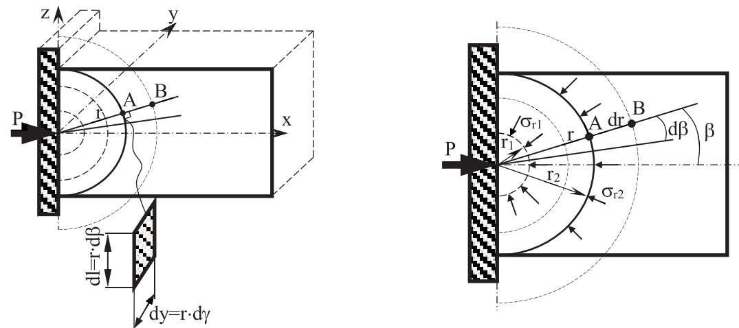
Рисунок 2 – Расчетная схема разрушения ударом частицы в форме бруса постоянного сечения
