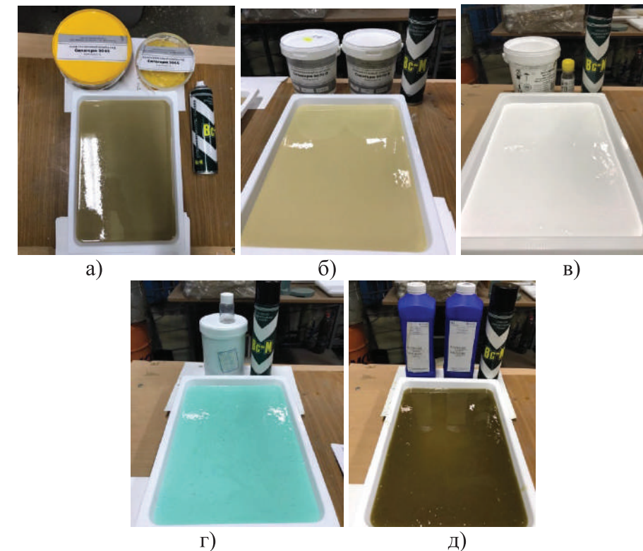
а – Силагерм 5045, б – Силагерм 6070П, в – Пентэласт 710, г – SilcoTin 40, д – PolyFlex 80
