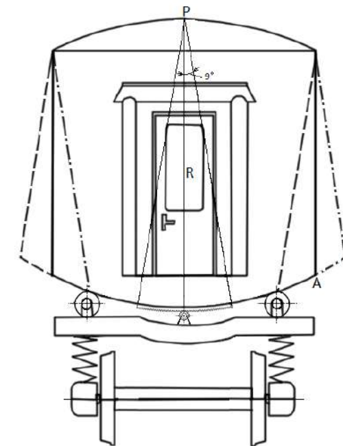
4-сурет – Көлбеу реттегіші бар жолаушылар вагоны: Р-вагонның полюсі (вагонның жоғарғы нүктесі); R-вагонның айналу шеңберінің радиусы (полюстен негізге дейінгі биіктік)
