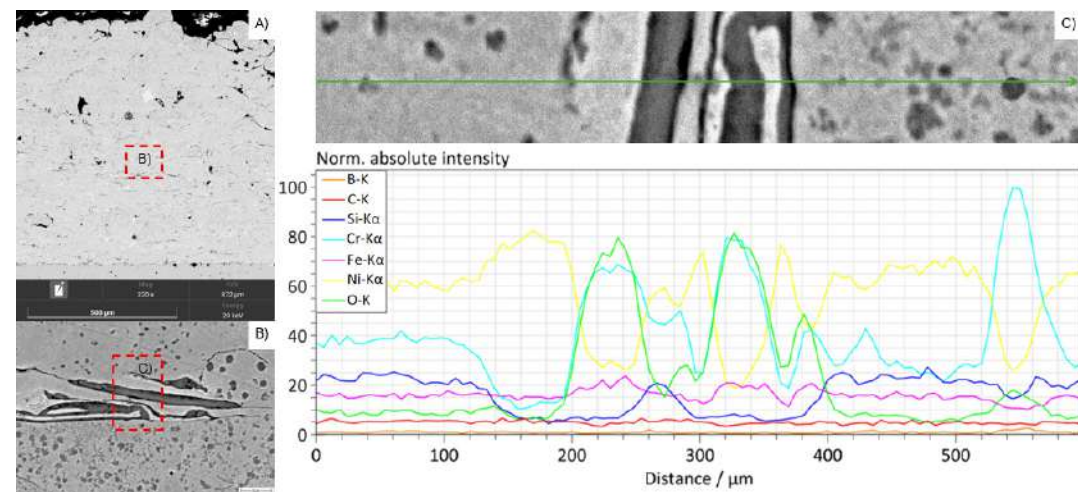
Рисунок 5 – Морфология покрытия после нагрева пистолетом для ГПН: а) общий вид покрытия б) морфология покрытия при увеличении \times 3000 с) линейный EDS анализ
