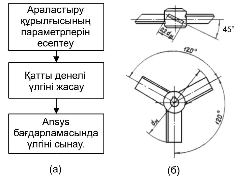
1-сурет – Эксперимент жүргізу схемасы (а), үш қалақшалы араластырғыштың параметрлері (б)
