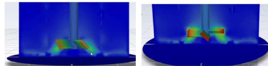
3-сурет – 60 айн/мин (а) және 90 айн/мин (б) жылдамдықтағы араластырғыш аппараттың қатты күйдегі моделі
