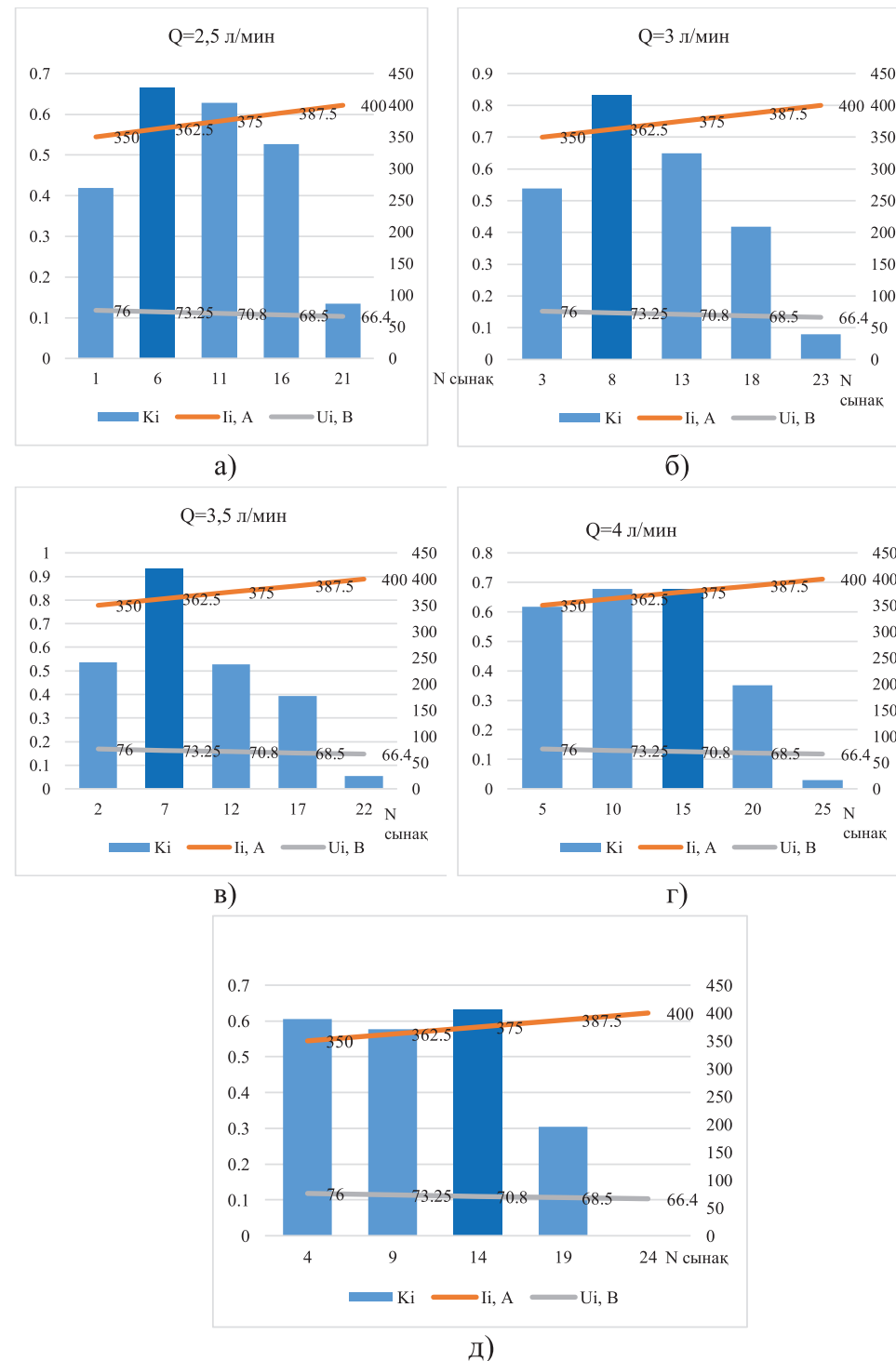
9-сурет – Кристаллизаторды салқындатуға жұмсалатын су көлемінің кешенді сапа көрсеткішіне әсері
