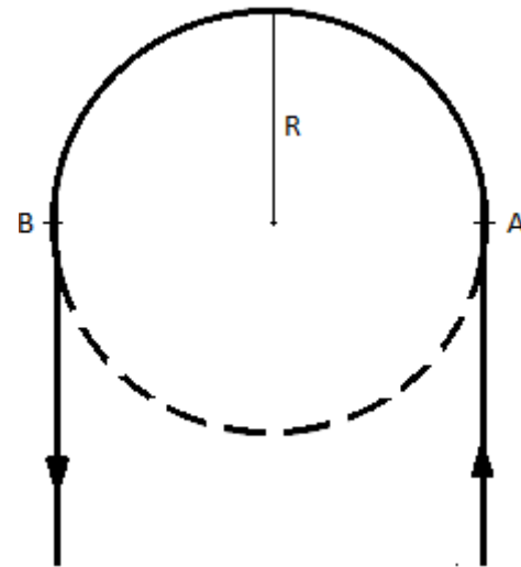
5-сурет – R=500 м радиусы бар қисықтағы жылжымалы құрамның қозғалысының сызбасы
