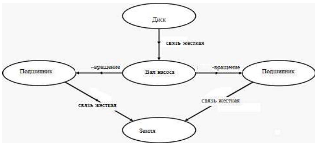
Рисунок 4 – Кинематическая схема ротора
