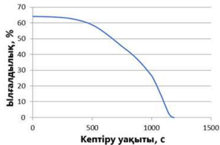
8-сурет – Экспресс-қыздыру кезінде алынған 2 % майлылығы сүзбені кептіру қисығы
