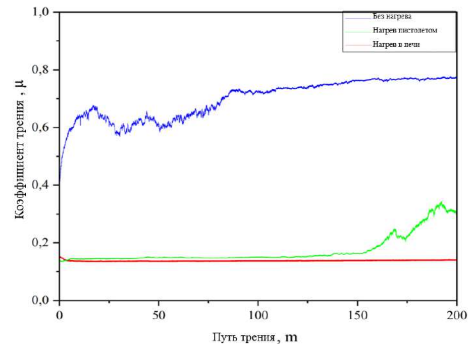
Рисунок 7 – Результаты трибологических испытаний
