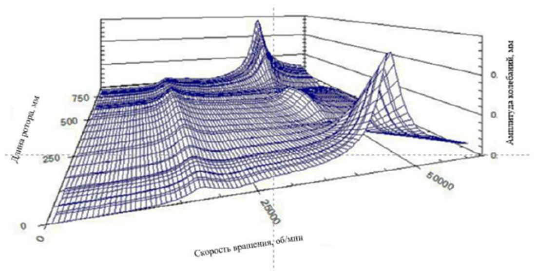
Рисунок 8 – Диаграмма АЧХ ротора
