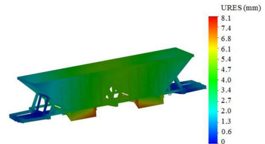
3-сурет – Хоппер вагонының түйіндеріндегі орын ауыстырулар
