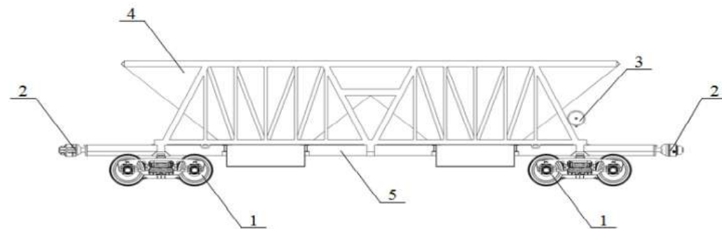
1-сурет– Екі секциялы хоппер вагон: 1 – шасси модулі; 2 – автоматты біріктіру модулі; 3 – тежеу жабдығының модулі; 4 – корпус модулі; 5 – жақтау (рама) модулі
