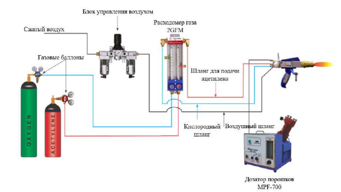
Рисунок 2 – Схема установки для газопламенного напыления
