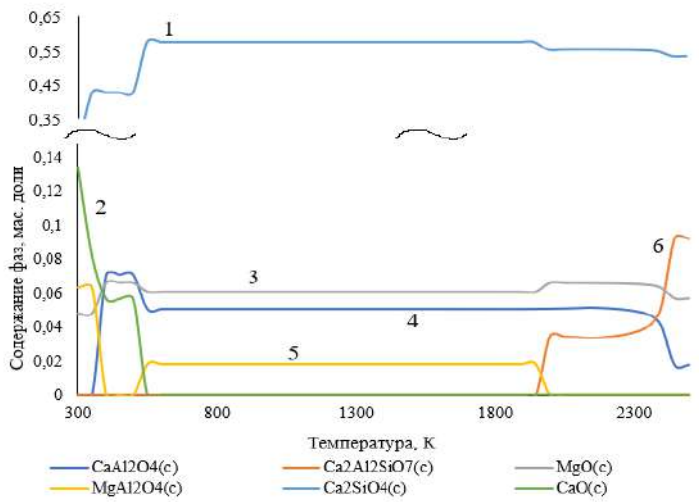
1 – Ca 2 SiO 4 ; 2 – CaO; 3 – MgO; 4 – CaAl 2 O 4 ; 5 – MgAl 2 O 4 ; 6 – Ca 2 Al 2 SiO 7 . Рисунок 1 – Динамика изменения фазового состава шлака с температурой по стандартной технологии
