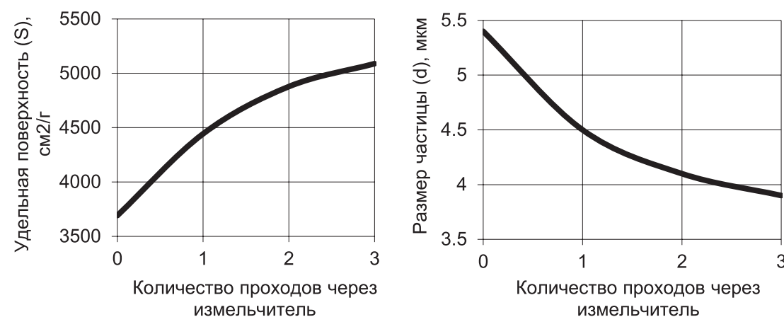
Рисунок 7 – Кинетика измельчения цемента в многоступенчатом измельчителе
