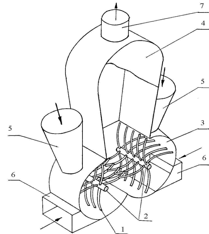
2-сурет – Полидисперсті материалдарды кептіруге арналған қондырғы:
