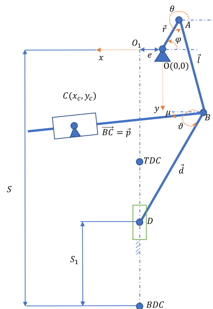
Рисунок 1 – кинематическая схема исполнительного механизма гибридного кривошипного пресса
