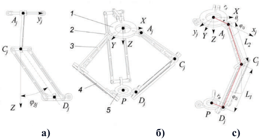
2 - сурет – Клавель дельта-роботының құрылымы: (а) негізгі көрініс, (б) бір аяқтың бөлек қарастырылуы, (с) Клавельдің дельта-роботының параметрлері
