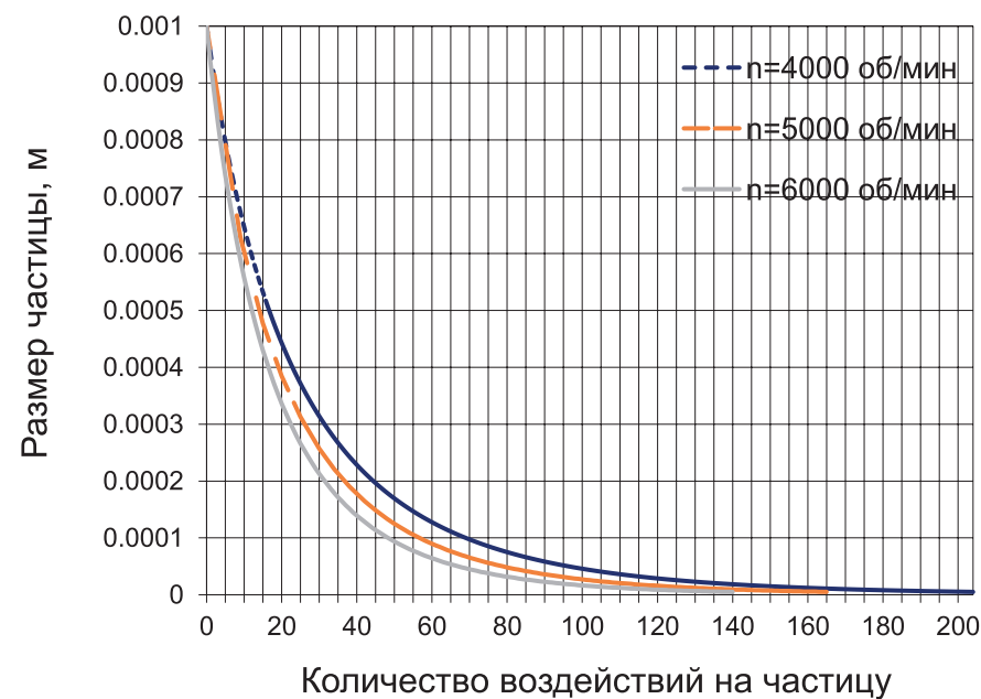
Рисунок 3 – Результаты расчета процесса измельчения частицы
