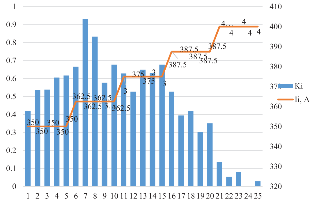
7 – сурет – Ток күшінің балқытылған тістер сапасының кешенді көрсеткішіне әсері
