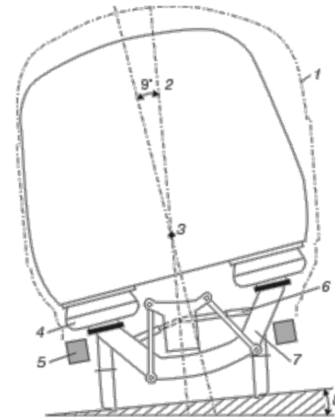
2-сурет – Вагон шанағының активті қисаю жүйесі бар пойыздың сызбасы:
