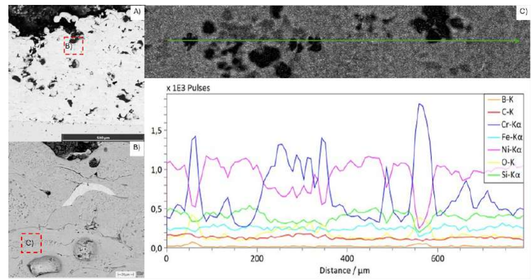
Рисунок 4 – Морфология покрытия без термического влияния: а) общий вид покрытия б) морфология покрытия при увеличении ×3000 с) линейный EDS анализ
