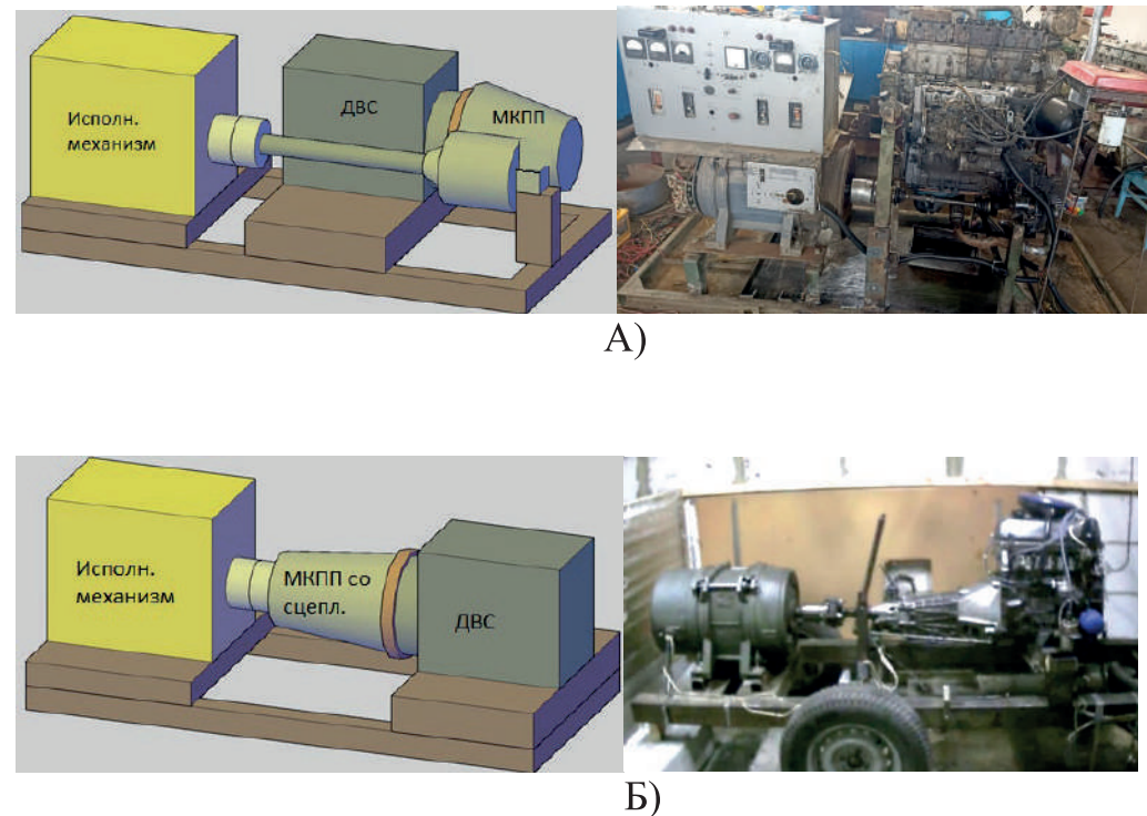
Рисунок 3 – Оборудование с приводом в сборе переднеприводной, и заднеприводной МКПП
