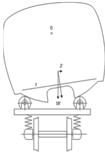
1-сурет – Вагон корпусының пассивті еңкею жүйесі бар 381 сериялы электр пойызының құрылымдық схемасы:
