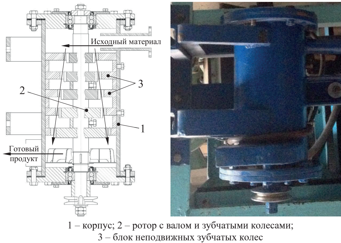
Рисунок 5 – Многоступенчатый измельчитель ударного действия
