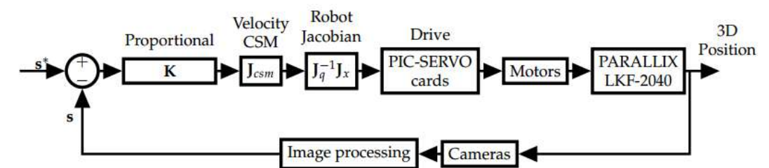
Рисунок 1 – Схема управления на основе скорости с помощью Camera Space Manipulation [15]
