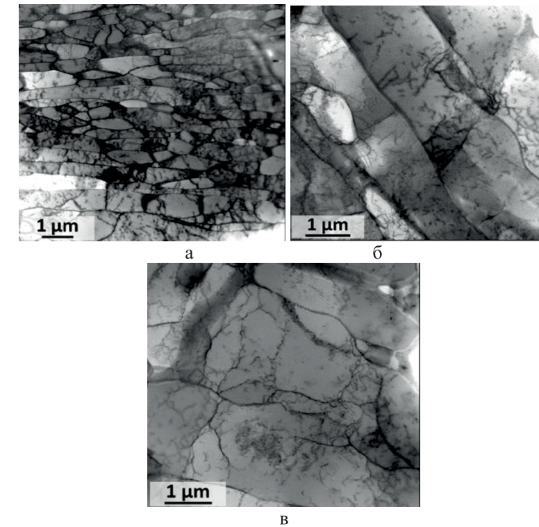
а – беттік қабат, б – ортаңғы қабат, в – орталық бөлік 2-сурет – Деформацияланған мыс сымның микроқұрылымы (көлденең қима)
