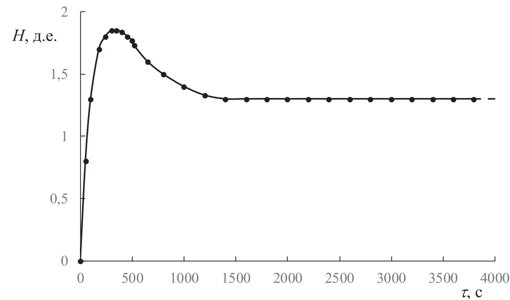
Рисунок 3 – Зависимость энтропии смешения фракций от продолжительности измельчения
