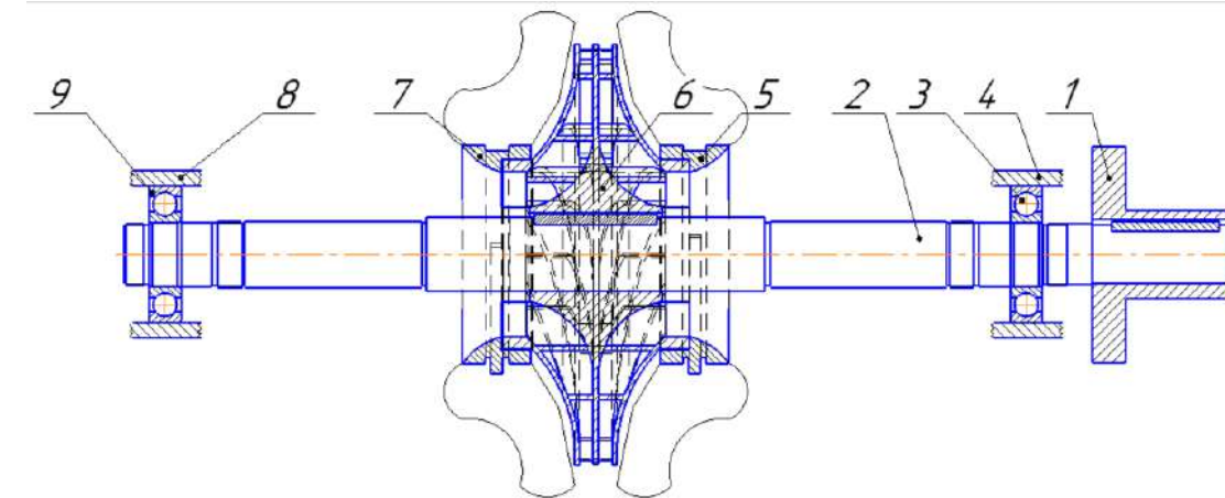
а) элементы насоса
