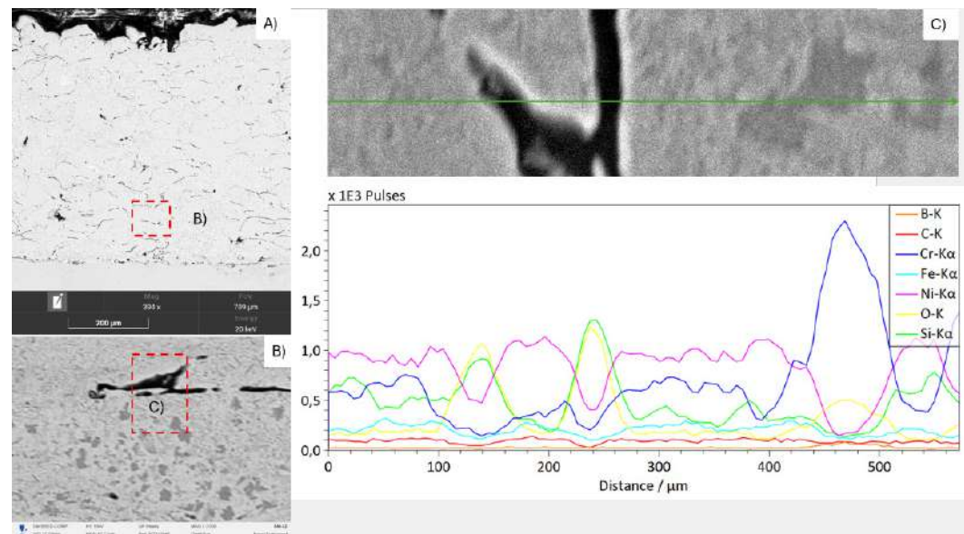
Рисунок 6 – Морфология покрытия после печи: а) общий вид покрытия б) морфология покрытия при увеличении \times 3000 с) линейный EDS анализ
