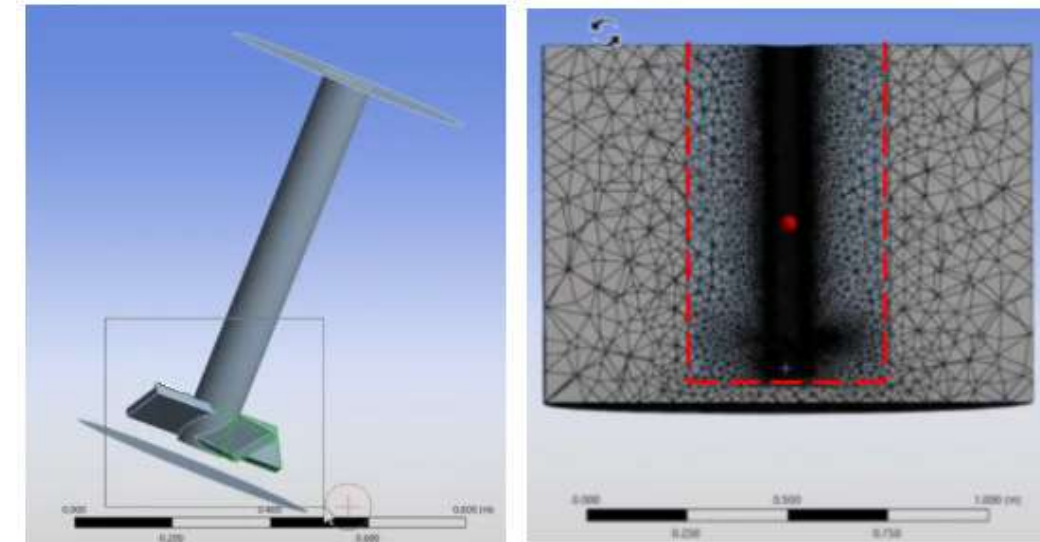
2-сурет – Араластырғыш аппараттың қатты күйдегі моделі (а) және соңғы элементтер торымен модель қимасы (б)
