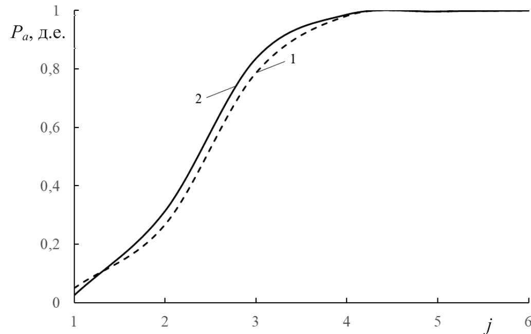
Рисунок 1 – Зависимость вероятности разрушения зерен от их размера по исходной P_a (17) – 1 и модифицированной P_a (18) – 2 моделям
