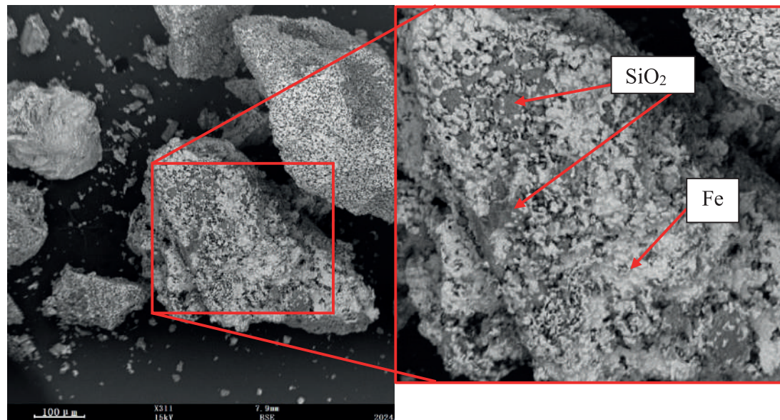
Рисунок 2 – РЭМ-изображение восстановленных частиц
