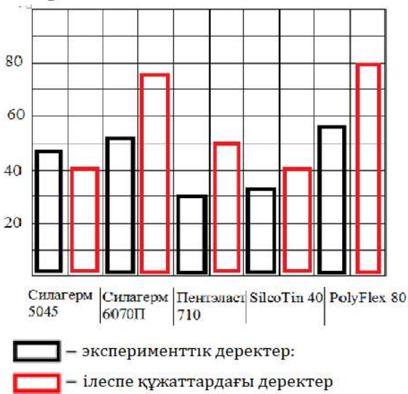
5-сурет – Өлшеу деректері мен ілеспе құжаттардағы мәліметтер бойынша Шор қаттылығының салыстырмалы диаграммасы
