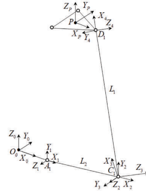
3 - сурет – Абсолюттік және жергілікті координаттар жүйелері
