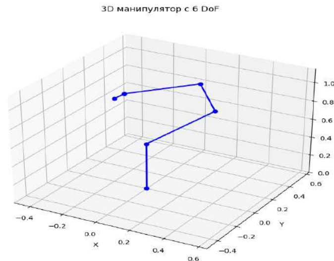
Рисунок 6 – Трехмерное моделирование траектории движения манипулятора
