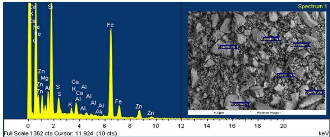
Рисунок 3 – Снимок, полученный с помощью растрового электронного микроскопа и микроанализ свинцового шлака при увеличении x500
