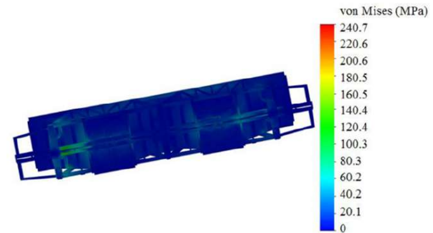
2-сурет – Хоппердің кернеулі күйі
