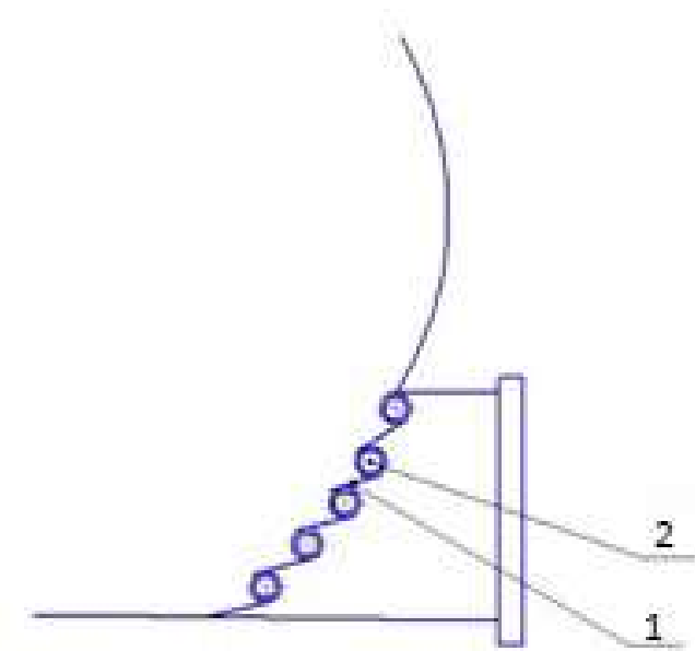
3-сурет – Полидисперсті материалдарға арналған кептіргіштің тангенциалды келтеқұбырлары: 1 – айналымы пластиналар; 2 – өс.
