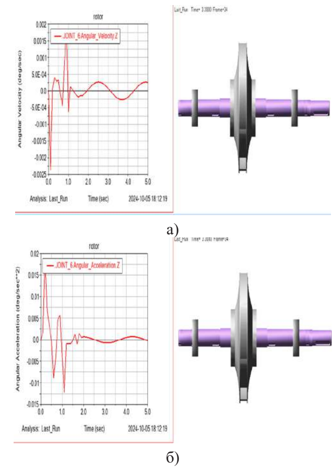
Рисунок 6 – Диаграммы изменений: а) скорости в подшипниковых опорах; б) ускорений в опорах
