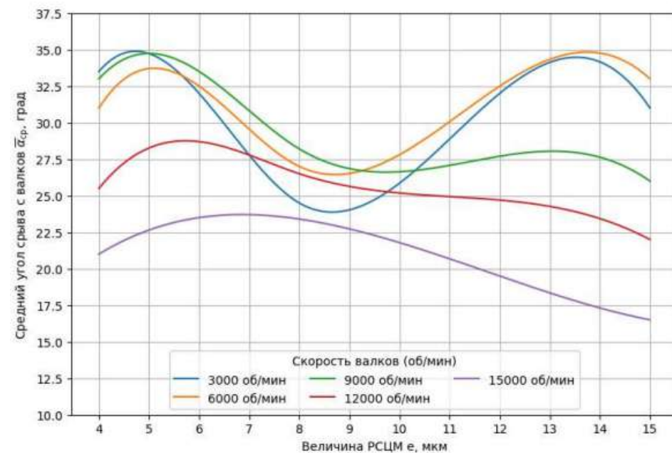
Рисунок 4 – Зависимость угла срыва от РСЦМ
