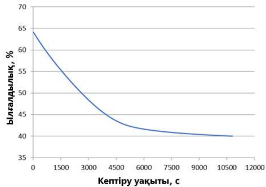
5-сурет – Майлылығы 2% сүзбені кептіру қисығы
