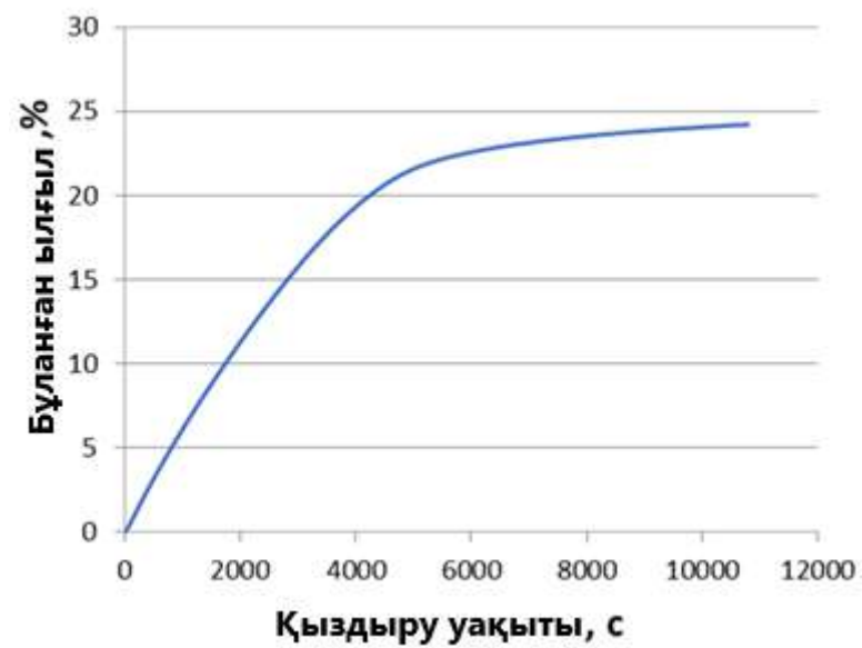
4-сурет – Кептіру процесінде 60°C температурада майлылығы 2 % сүзбеден ылғалдың булануы
