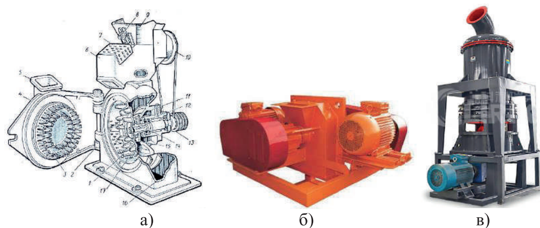
Рисунок 1 – Измельчители ударного действия: аэробильная мельница (а), дезинтегратор (б), центробежная мельница (в)
