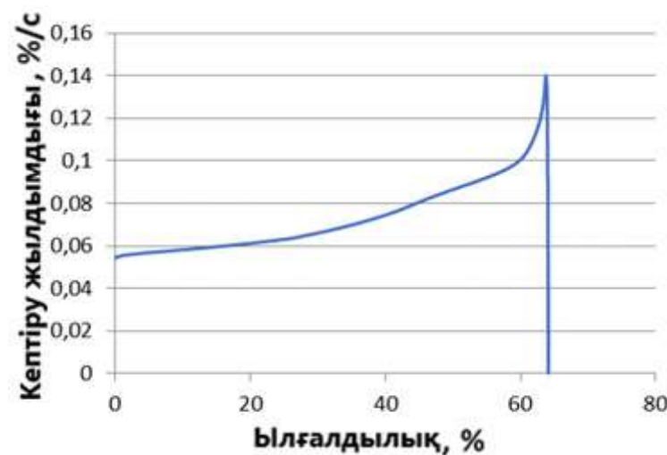
9-сурет – Экспресс-қыздыру кезінде алынған майлылығы 2 % сүзбені кептіру жылдамдығының қисығы
