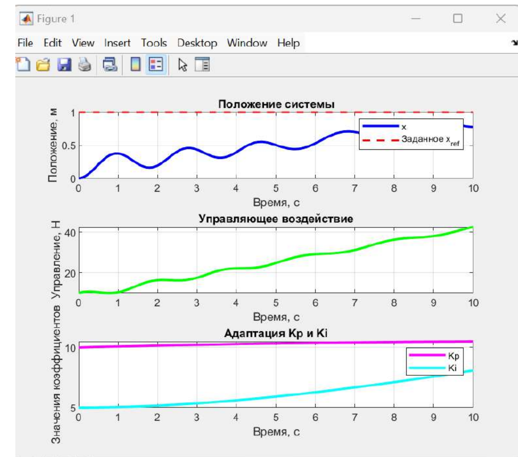
Рисунок 3 – Положение системы, управляющие воздействие и коэффициенты адаптации
