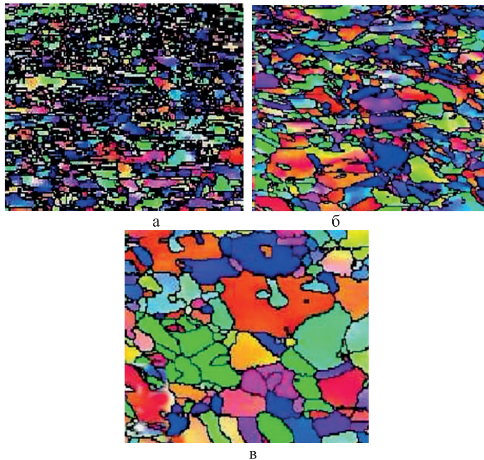
а – беттік қабат, б – ортаңғы қабат, в – орталық бөлік 3-сурет – Деформацияланған мыс сымның микроқұрылымының бағдарлану карталары (көлденең қимасы)
