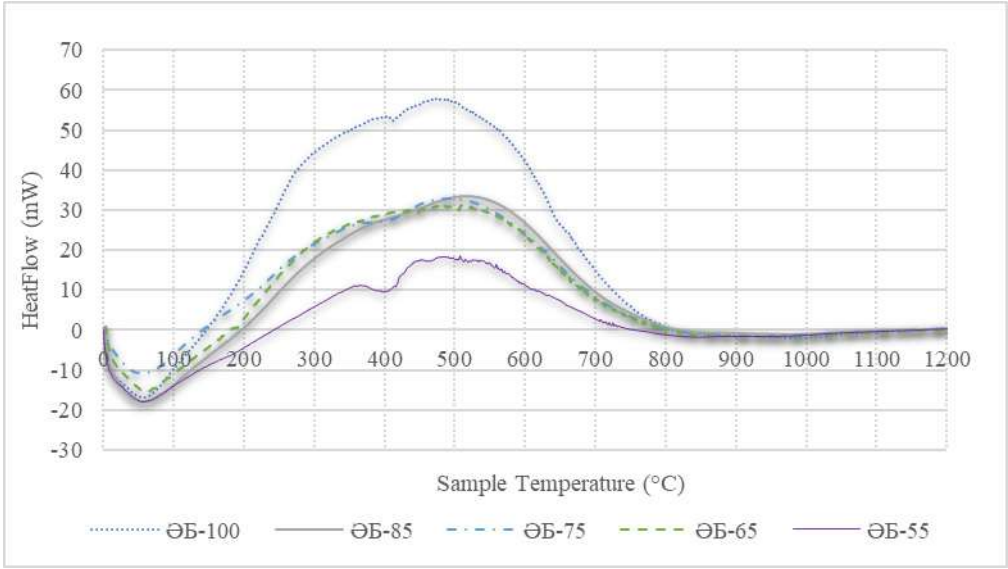
2-сурет – Зерттелетін көмірдің жылу әсері
