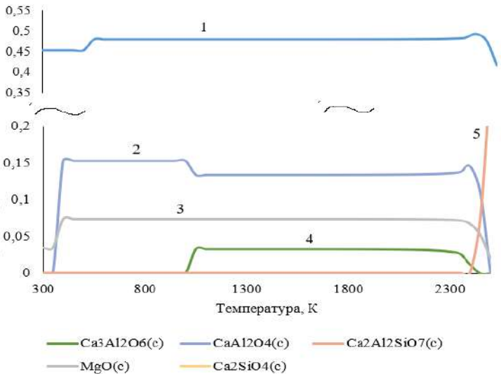
1 – Ca 2 SiO 4 ; 2 – CaAl 2 O 4 ; 3 – MgO; 4 – Ca 3 Al 2 O 6 ; 5 – Ca 2 Al 2 SiO 7 . Рисунок 2 – Динамика изменения фазового состава шлака с температурой с применением ФАСК
