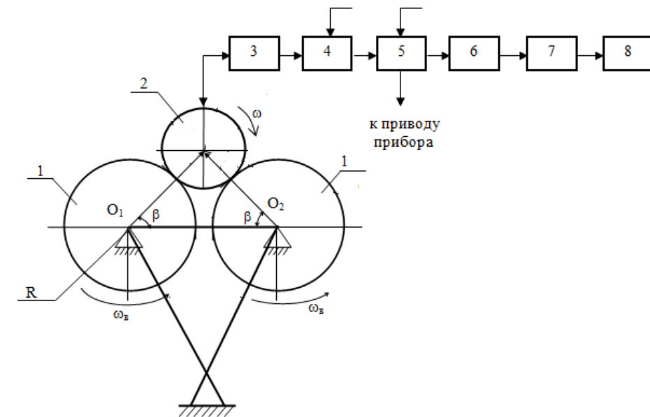
Рисунок 1 – Функциональная схема прибора
