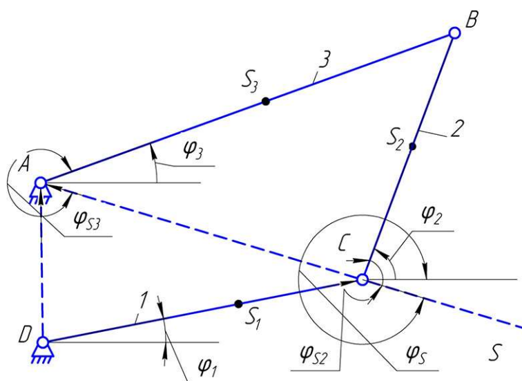
Рисунок 3 – Кинематический анализ механизма подъема и спуска робота-спутника
