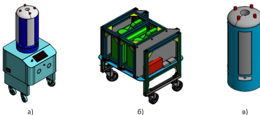
а) общий вид, б) нижняя часть робота для жидкой дезинфекции, в) верхняя часть робота, предназначенная для УФ дезинфекции и для работы в режиме рециркулятора
