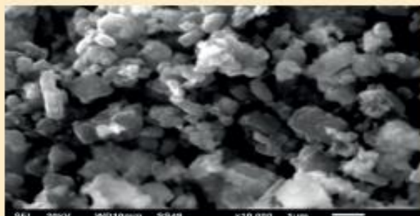
Рис. 3. Микрофотография адсорбента на основе цеолита, модифицированного ксерогелем оксида ванадия и титана.
