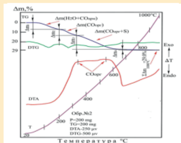
Рис. 2. Дериватограмма цеолита, модифицированного гибридной композицией оксидов ванадия и титана.
