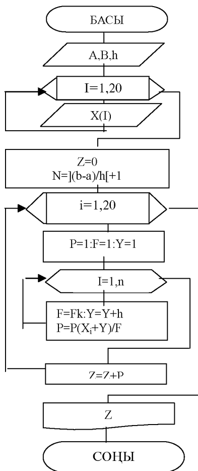
1.8.3-сурет.Есептің блок-схемасы
