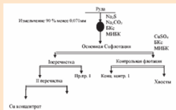
Рис. 5. Схема флотации медно-золотосодержащей руды месторождения Коктасжал.
